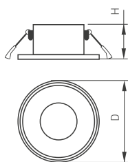
Рис. 1. Чертеж и габаритные размеры
